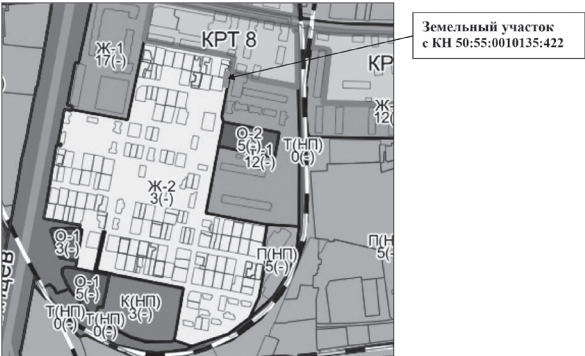
Рисунок 1 – Фрагмент карты градостроительного зонирования
