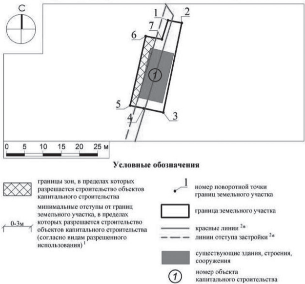
Рисунок 2 – Чертеж градостроительного плана земельного участка
