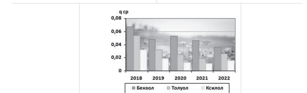
Рисунок 2.2.1 – Тенденция среднегодовых концентраций бенз(а)пирена (*10-6 мг/м3), взвешенных веществ, хлорида водорода, бензола, ксилола, толуола (мг/м3) за период 2018-2022 гг. в г. Подольске
